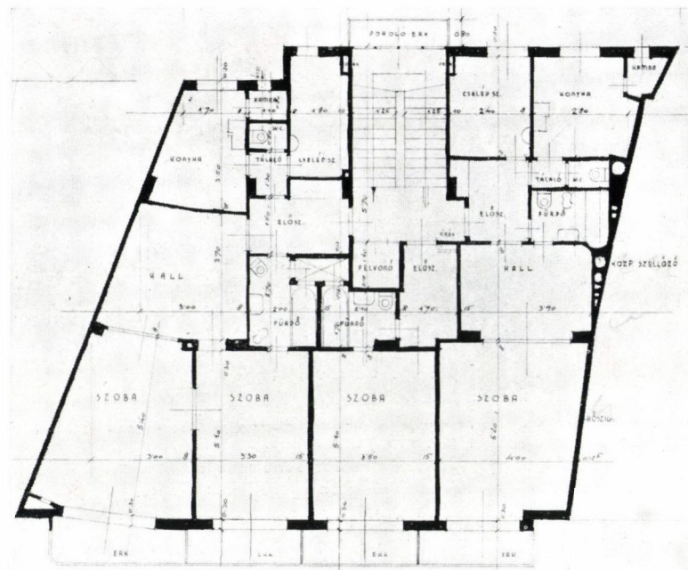
Bérház a Margit-körúton — Tervezte: Preisich és Va- dász — A felső alaprajz a Margit-körúti, az alsó a Írók körúti bérház általános emeleti alaprajza.
