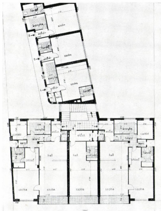
Travertin homlokzatú bérház Budapesten, a Szépcsútcában — Tervezték: Lauber és Nyiry — Miethaus in Budapest — Façade mit Travertin verkleidet — Kivitel: Havel Lipót — Ablaksor Koszmoport-rendszerü — Borsos felv. — Jobboldalt: Előcsarnok, műmárvány burkolással — Világítás Holitscher Zsigmond és Tsa Ludvig felv.
