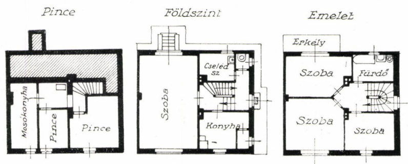
Saroktípus
