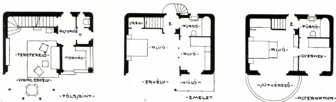
Kis családi ház terve
